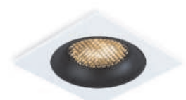
TN102727 белый, черный 92*92*23 Ø80 GU5.3*1 max 12W IP20
