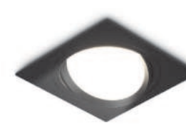
TN51917 черный 115*115*23 Ø98 GX53*1 max 12W IP20
