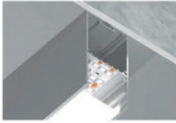
GP3000AL серебро, матовый 2000*35*67 мм Алюминиевый профиль накл./подв. Profile System для ленты до 32,8мм 4 420 р.
