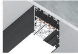
GP3050BK черный, матовый 2000*42*45 мм Алюминиевый профиль накл./подв. Profile System для ленты до 33,4мм 5 160 р.
