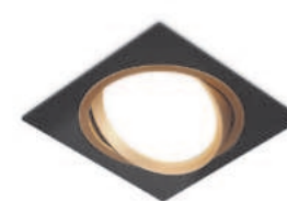
TN51918 черный, золото 115*115*23 Ø98 GX53*1 max 12W IP20
