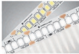
GS3502 белый 5000*10*1.2 LED 22 Вт/мW IP20 4500K дневной белый свет 3 120 р.
