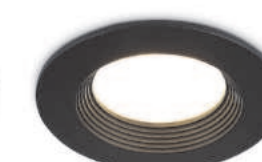
TN102816 черный D80*28 Ø70 GU5.3*1 IP20
