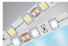
GS4003 белый 5000*10*1.87 LED 14.4 Вт/мW IP20 6500K холодный белый свет 1 170 р.
