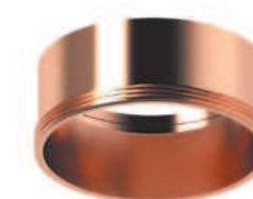
N6114 золото розовое полированное D60*30 GU5.3*1 max 10W IP20
