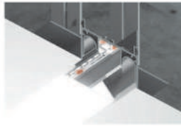
GP4000AL серебро, матовый 2000*72.2*34 мм Алюминиевый профиль под натяж. потолок для ленты до 13.2мм 3 370 р.
