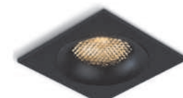
TN102729 черный 92*92*23 Ø80 GU5.3*1 max 12W IP20
