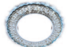
G315 CL/CLD хром D125*25 Ø87 GX53 IP20 3W 6400K 640 p.
