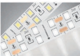
GS3602 белый 5000*14*1.2 LED 20 Вт/мW IP20 4500K дневной белый свет 2 750 р.
