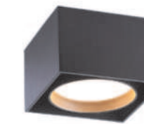
TN70866 черный 95*95*62 GX53*1 max 12W IP20
