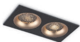
TN102735 черный, золото 175*92*23 Ø160*80 GU5.3*2 max 12W IP20
