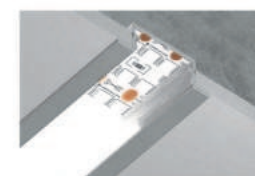
GP1200AL серебро, матовый 2000*28.6*10 мм Алюминиевый профиль встраиваемый для ленты до 18,5мм 960 р.
