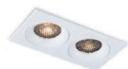
TN102731 белый 175*92*23 Ø160*80 GU5.3*2 max 12W IP20
