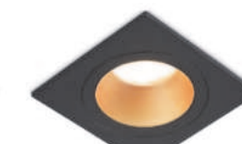
TN102829 черный, золото 92*92*50 Ø70 GU5.3*1 IP20
