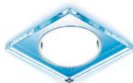
G215 CL/CH/CLD прозрачный, хром D120*120*22 Ø87 GX53*1 max 12W IP20 3W 6400K 640 p.
