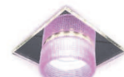
TN356 хром, прозрачный 95*95*45 Ø60 Ø60*60 GU5.3*1 max 10W IP20 3W 6400K
