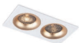
TN102733 белый, золото 175*92*23 Ø160*80 GU5.3*2 max 12W IP20
