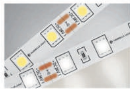
GS4002 белый 5000*10*1.87 LED 14.4 Вт/мW IP20 4500K дневной белый свет 1 170 р.
