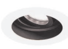
TN176 белый, черный D100*40 Ø92 GU5.3*1 max 12W IP20
