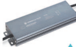
GS9865 серебро 220*65*28 LED 200W IP67 Блок питания 3 710 р.
