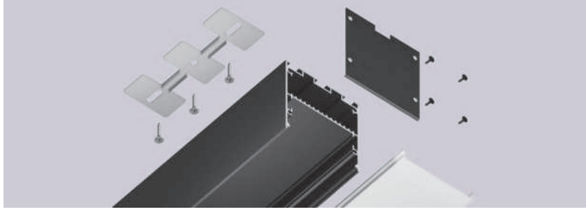
GP3000BK черный, матовый 2000*35*67 мм Алюминиевый профиль накл./подв. Profile System для ленты до 32,8мм 4 870 р.
