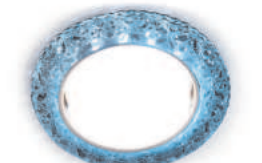
G308 CL/CLD прозрачный, хром D120*25 Ø87 GX53*1 max 12W IP20 3W 6400K 640 p.
